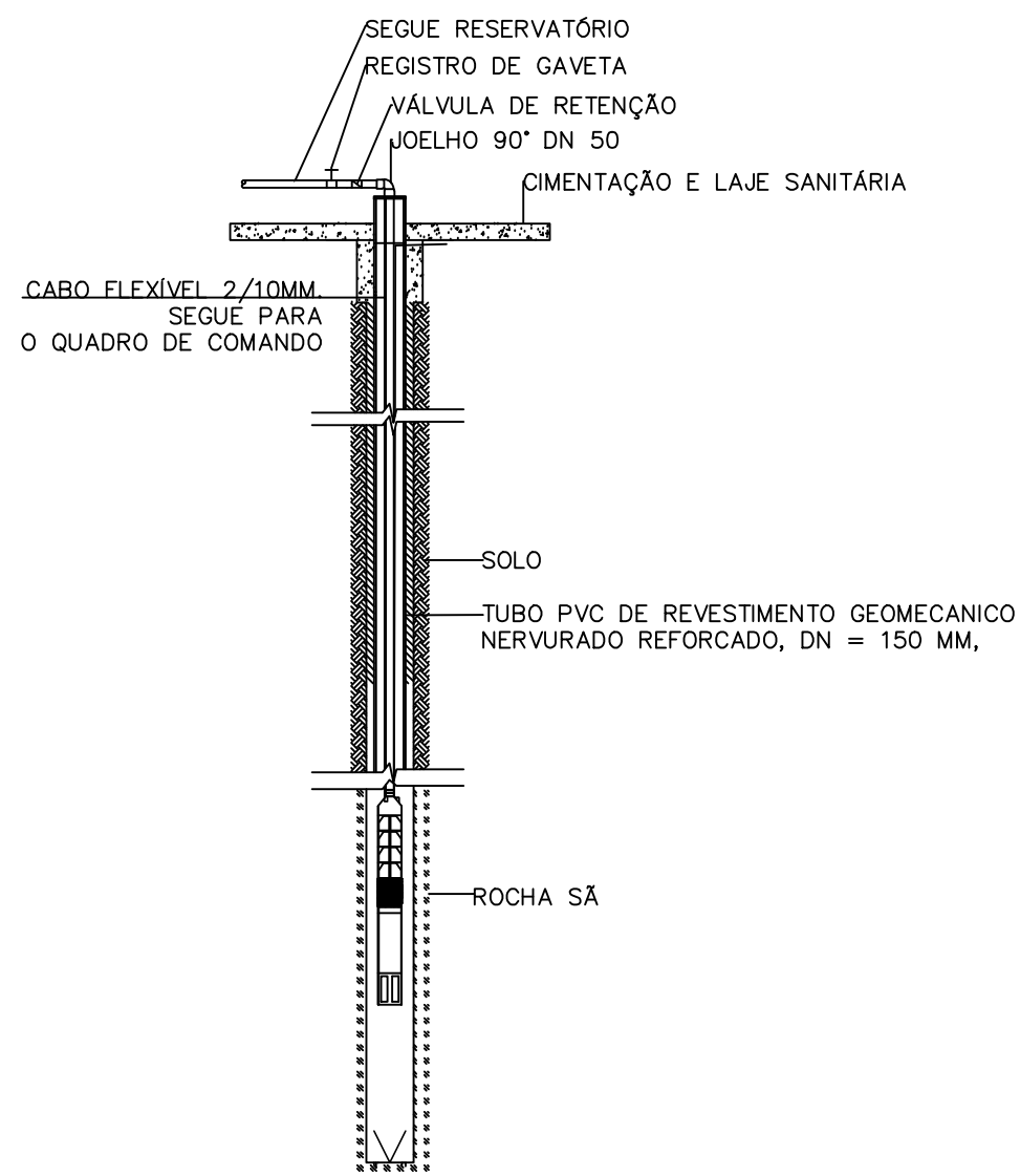
DETALHE CONSTRUTIVO DO POÇO
